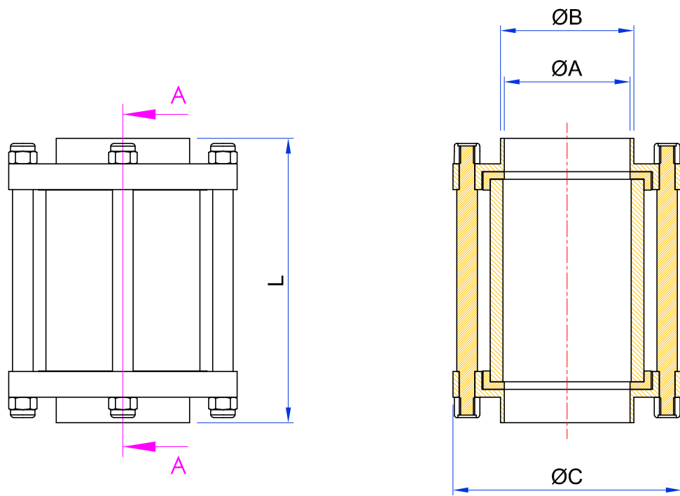
SEZIONE A-A
